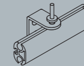
Haltewinkel mit Spannschraube M4 und Rändelmutter, Art.-Nr.: 8880014
