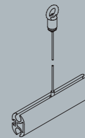
Öse mit Klemme und Seil 1,5 mm, Seillänge 500 mm*, Art.-Nr.: 8880001
