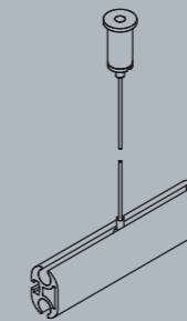
Boden-/Deckenanker Seilklemme und Seil 1,5 mm, Seillänge 500 mm*, Art.-Nr.: 8880005
